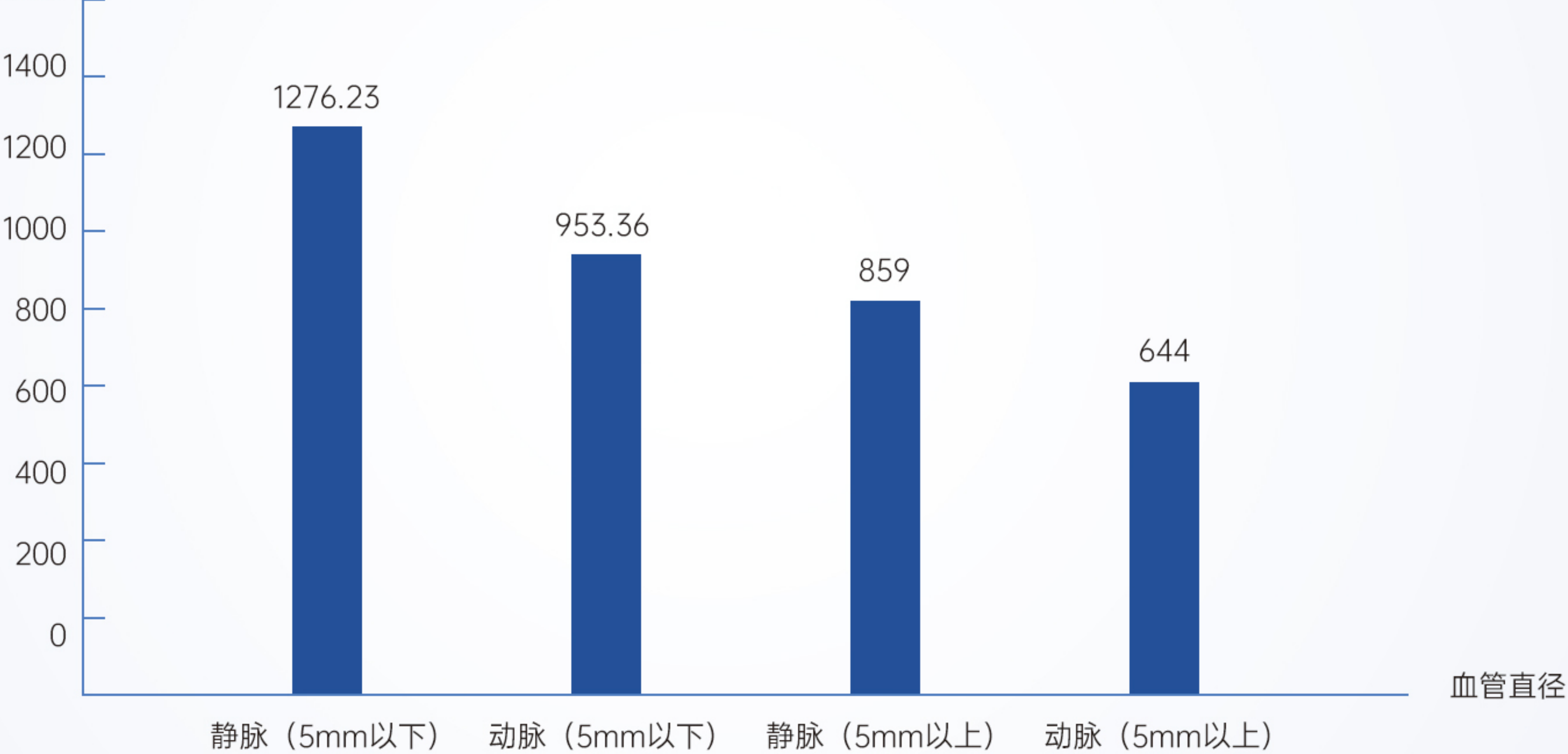
血管爆破压实验
